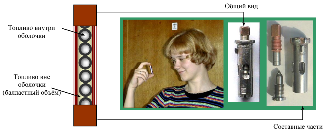
Рис. 5. Мишенный контейнер с заполненными D_2 -топливом оболочками (разработано в ФИАН при построении мишенной системы в рамках проекта МНТЦ № 512)
