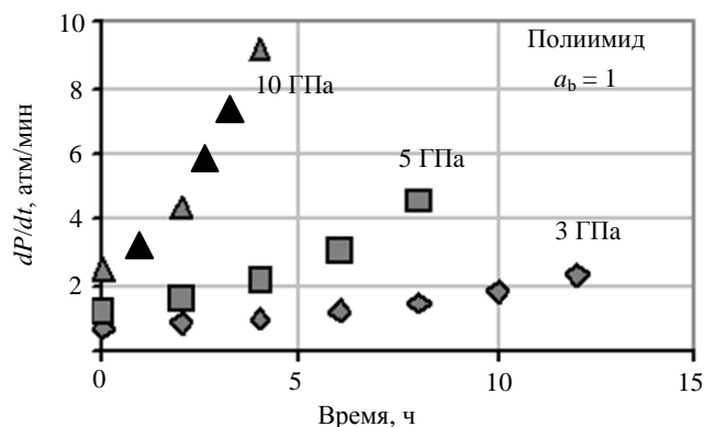
Рис. 9. Скорость заполнения как функция времени при различных значениях прочности оболочки ( D_2 , 1000 атм, 300 К)
