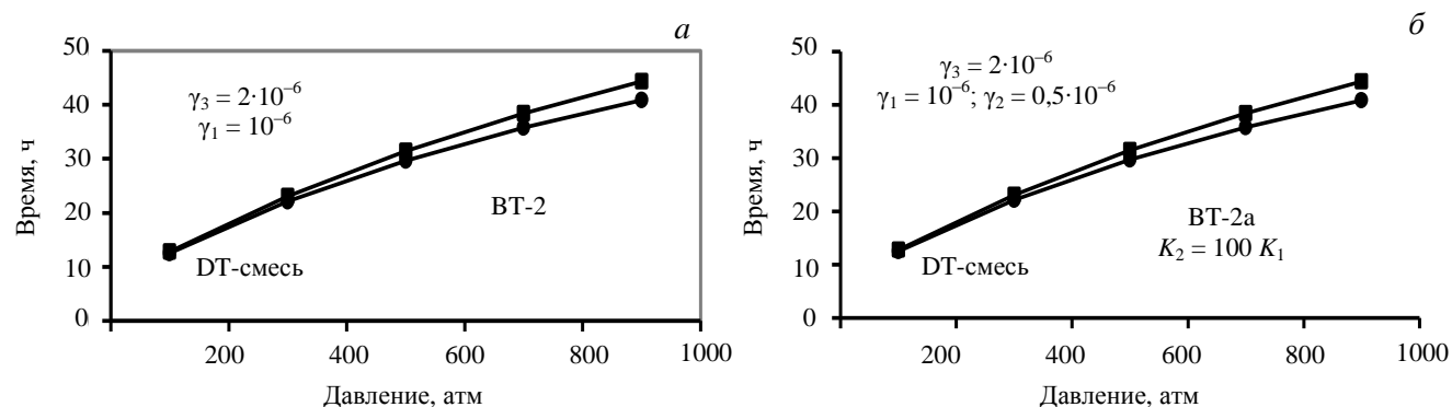
Рис. 2. Влияние радиационных дефектов на ход процесса заполнения для мишеней ВТ-2 и ВТ-2а
