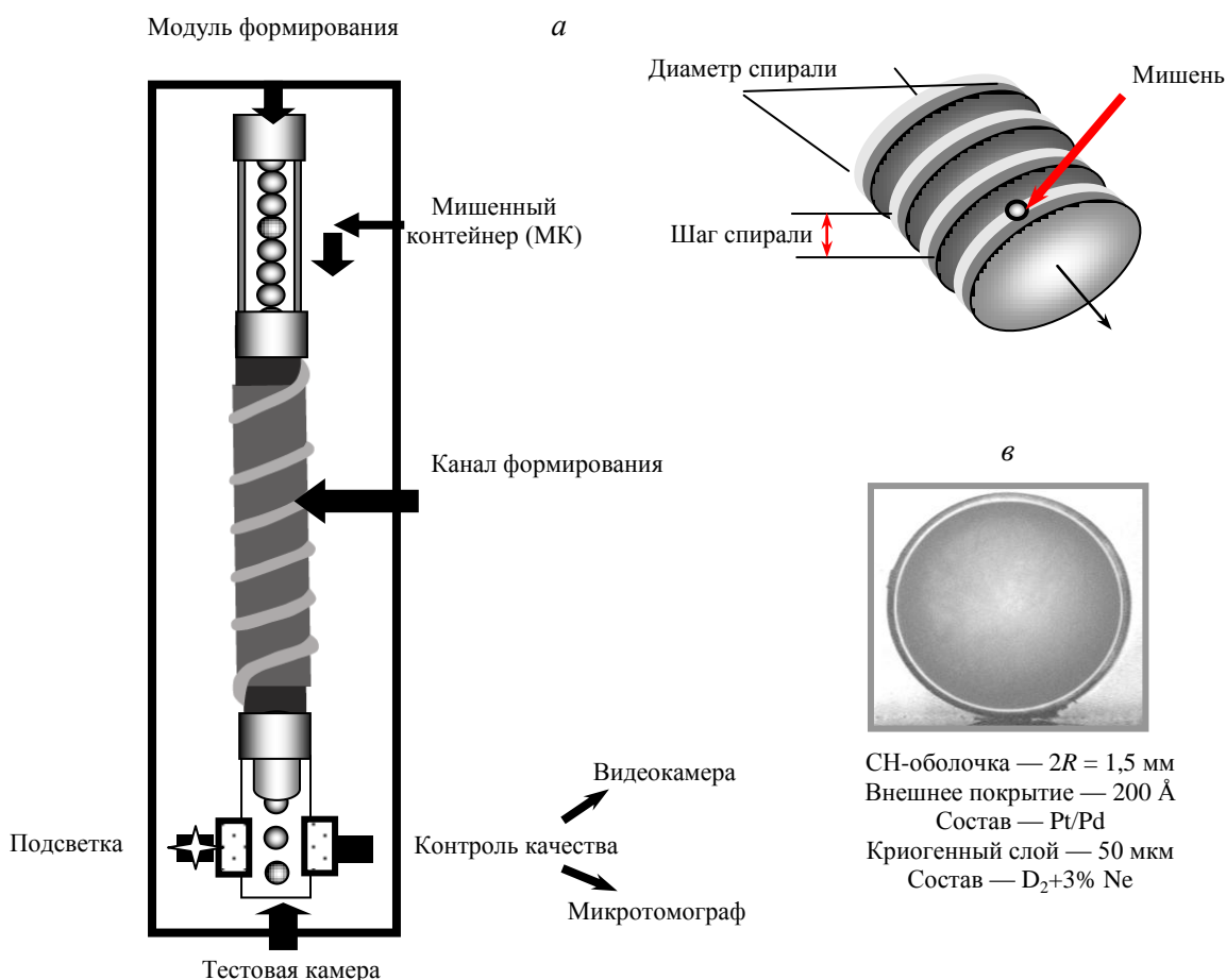
Рис. 12. Непрерывное формирование бесподвесных мишеней методом FST: а — схема модуля формирования; б — движение мишени по спиральному каналу формирования; в — сформированная в канале мишень
