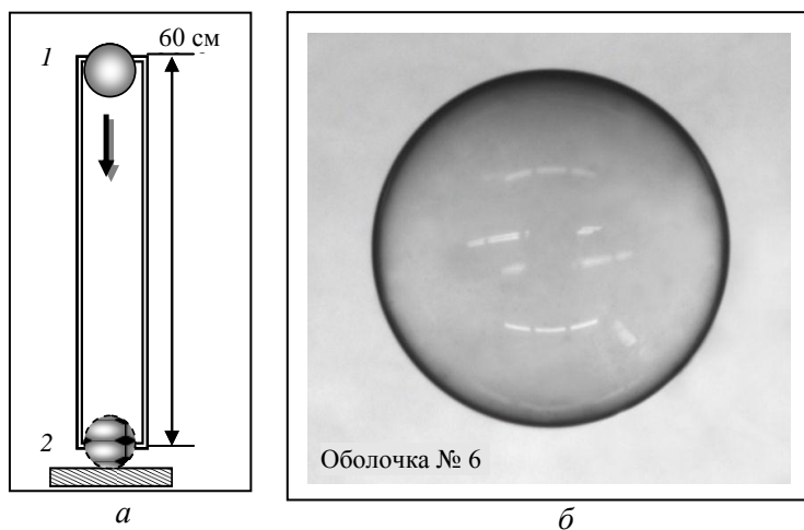
Рис. 14. Проброс оболочек из материала ПАМС в вертикальном канале: а — схема эксперимента; б — оболочка после её приземления (положение 2 на рисунке а). Параметры оболочки: \varnothing 1862 мм, толщина стенки 19,8 мкм, вес 231,3 мкг
