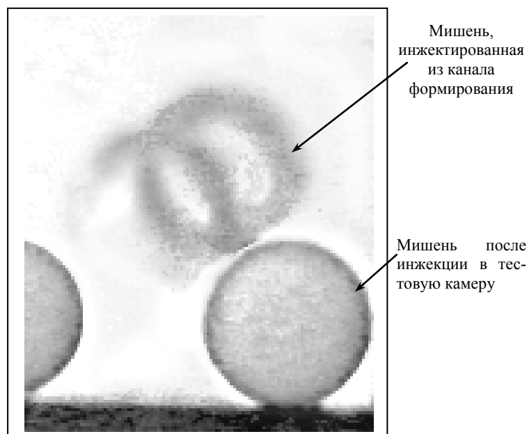
Рис. 13. Инжекция мишеней из канала формирования в оптическую тестовую камеру при T = 4,2 К
