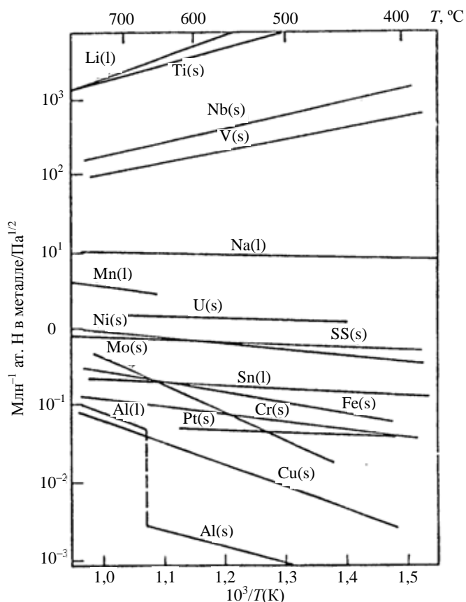
Рис. 16. Растворимость водорода в металлах и сплавах в зависимости от температуры [30]
