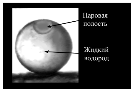
Рис. 7. СН-оболочка ( \varnothing 996 мкм) заполнена H_2 до 1000 атм при 300 К, а затем охлаждена до 32 К
