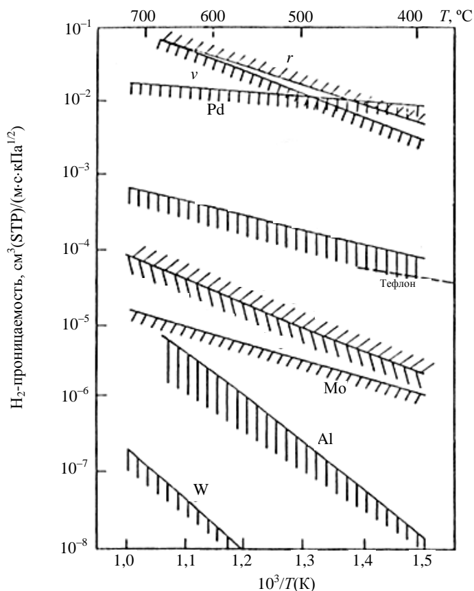
Рис. 17. Водородная проникаемость металлов и сплавов в зависимости от температуры [30]; STP — стандартное давление
