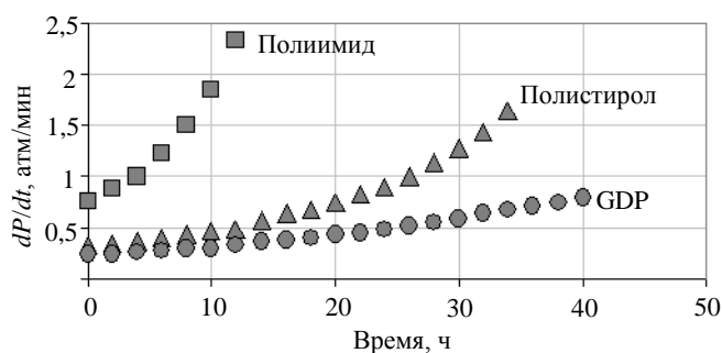
Рис. 8. Управляющая кривая, или скорость заполнения как функция времени для трёх различных материалов оболочки: полиимид, полистирол и GDP-полимер ( D_2 , 1000 атм, 300 К)
