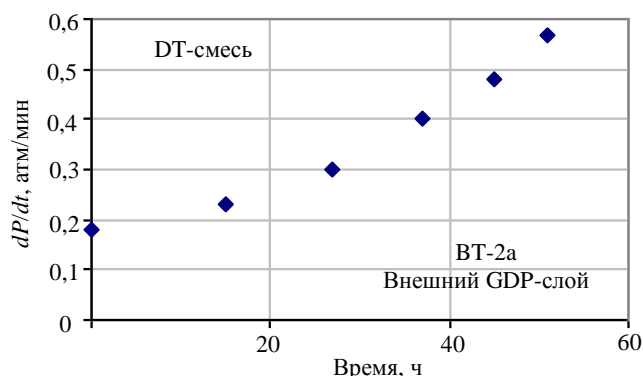
Рис. 4. Скорость заполнения как функция времени (1000 атм, DT при 300 К)
