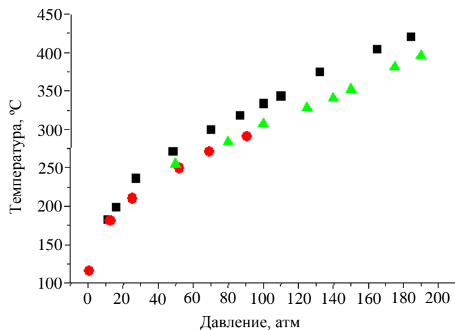
Рис. 15. Температурная зависимость давления термодиссоциации в области плато [28]: ■ — H 2 ; ● — D 2 ; ▲ — H 2 -D 2
