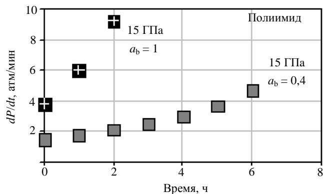
Рис. 10. Скорость заполнения как функция времени при различных значениях коэффициента запаса ( D_2 , 1000 атм, 300 К)
