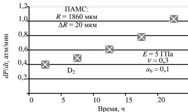
Рис. 11. Скорость заполнения как функция времени (1000 атм, D_2 )
